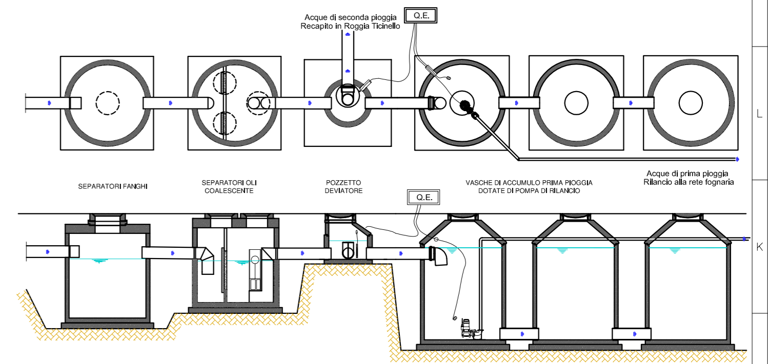
PARTICOLARE IMPIANTO DI TRATTAMENTO ACQUE
